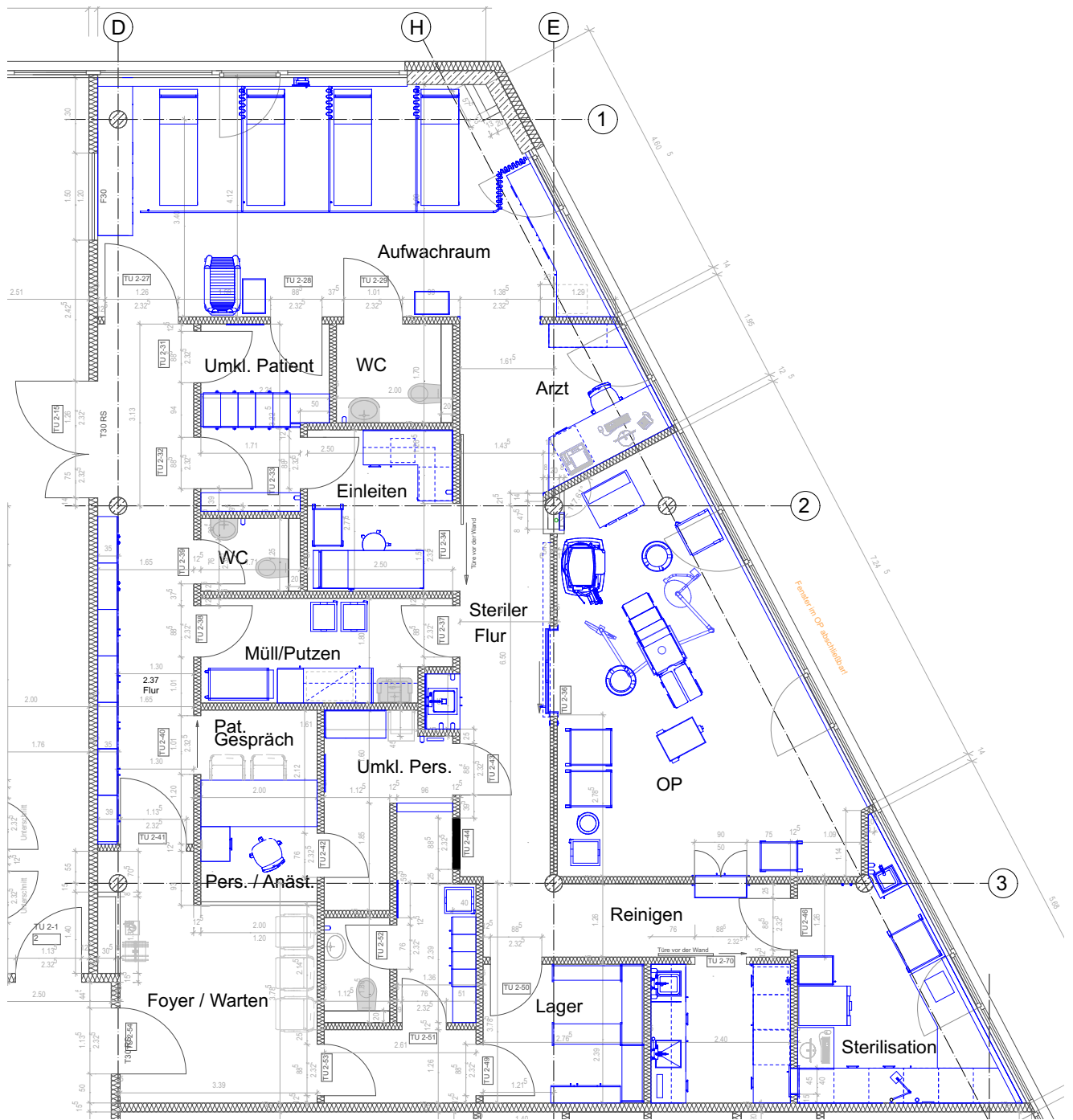
Grundriss
